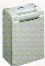
A034 DESKSIDE SHREDDERS 碎紙機 型號 20090 PSe 20092 PSeC 納紙寬度 240mm 240mm 紙屑尺寸 3.9mm 2 X 28mm 操控 自動 自動 體積(mm) 455 X 418 X 270 455 X 418 X 270 型號 20100 PS 20112 PSC 納紙寬度 240mm 240mm 紙屑尺寸 3.9mm 2 X 28mm 操控 自動 自動 體積(mm) 520 X 390 X 300 520 X 390 X 300
